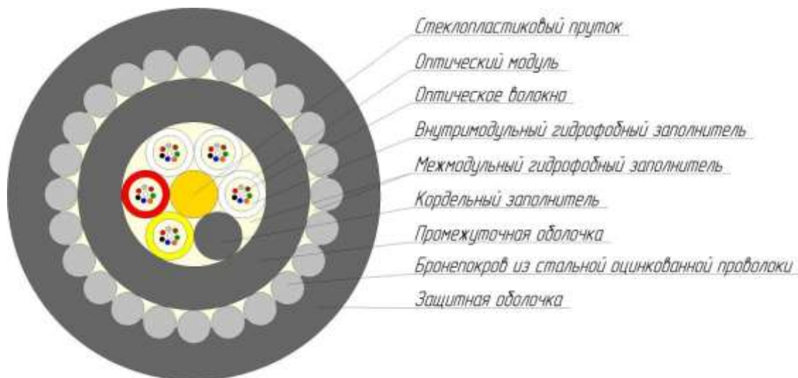
Кабель ОКБ-0,22-34...48П 7кН
